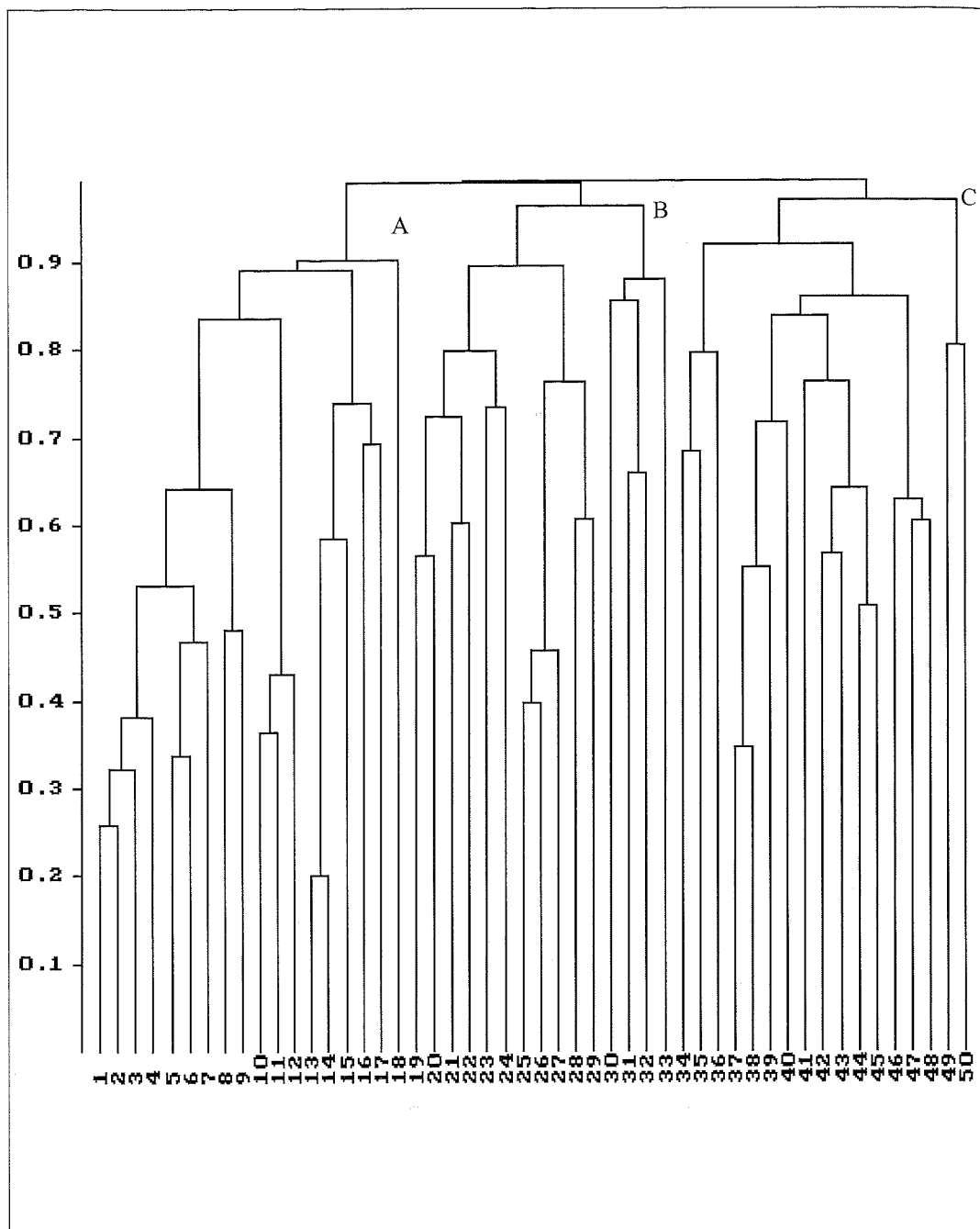
FIGURA 1. Clasificación mediante razón de similitud y vinculación completa. Classification by Similarity Ratio and Complete Linkage.
