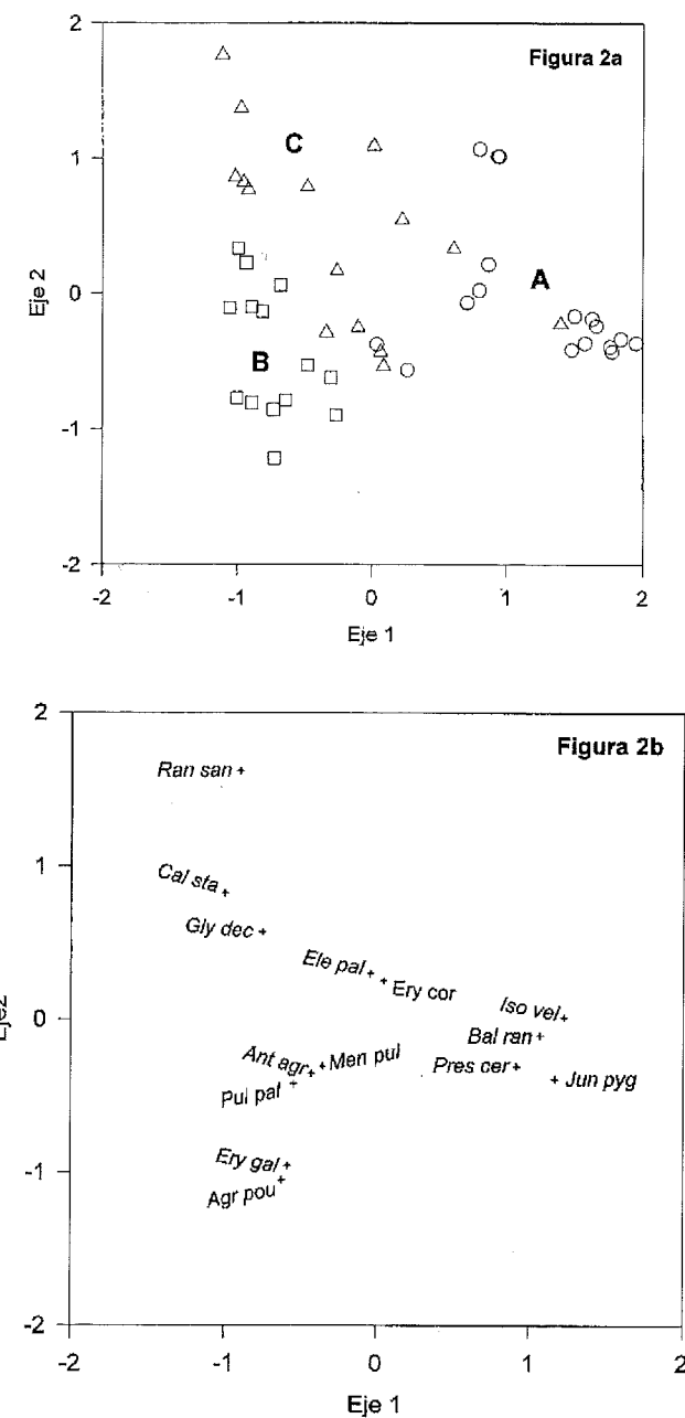
FIGURA 2. Ordenación mediante análisis de correspondencias de localidades (2a) y de especies (2b). Grupo A, círculos; grupo B, cuadrados; grupo C, triángulos. Ordination by Correspondence Analysis of localities (2a) and species (2b). Group A, circles; group B, squares; group C, triangles.
